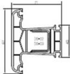
PRDR03 Orta Kayıt Profili Mullion Profile
