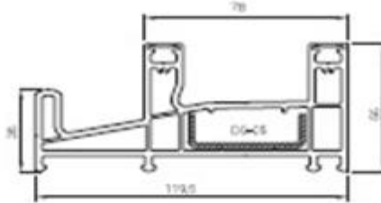
PRSY47 Sineklikli Kasa Profili Frame Fly Screen Profile
