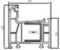
PRVN01 Kasa Profili Frame Profile
