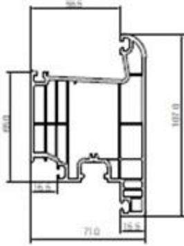
PRSC05 3 Contalı Dışa Açılım Kapı Profili Triple seal Outside Opening Door Profile
