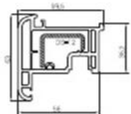
PR7113 Hareketli Orta Kayıt Profili Overhang (Stump)
