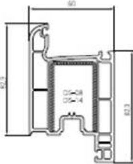
PRVN04 Kilitli Kapı Profili Door Sash Profile
