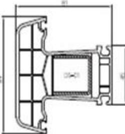
PRGR03 Orta Kayıt Profili Mullion Profile
