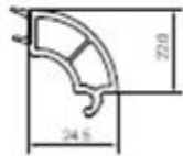
PRSC19 24 mm Cam Çıtası 24 mm Glazing Bead
