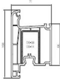
PR7105 Dışa Açılım Kapı Profili Outside Opening Door Profile
