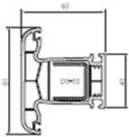
PRVN03 Orta Kayıt Profili Mullion Profile
