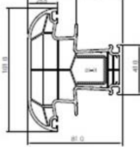
PRSC03 Orta Kayıt Profili Mullion Profile
