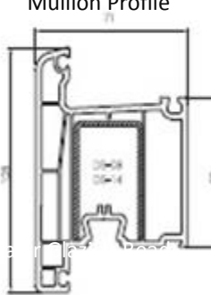
PR7113 Hareketli Orta Kayıt Profili Overhang (Stump) Çıtalar Glazing Bead
