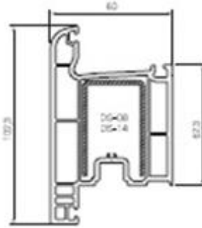
PRVN05 Dışa Açılım Kanat Profili Outside Opening Sash Profile
