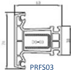
PRFS03 Orta Kayıt Profili Mullion Profile
